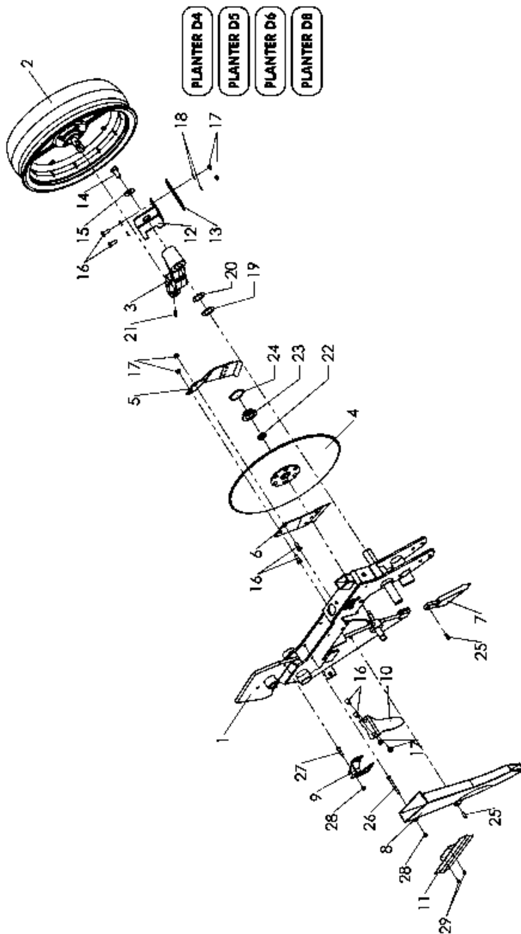
Pneumatic disc coupler seed drill sowing group-A, Diskli pnomatik mibzer ekim grubu-A, Группа сошника с дисковым сошником-A
